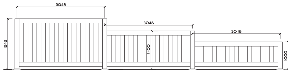
2 WOOD SCREEN FENCE STEP DOWN L07 SCALE: N.T.S.
